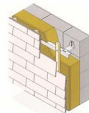
Hinterlüftete Fassade
