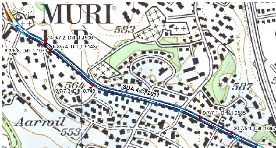
Abbildung 9: Veranschaulichungsbeispiel Homogenitätsanalyse SNHT auf dem SDA 4 C Belag in Muri. Breakpoints (rot), jeweils mit Ergebnis des T-Tests, sowie der Differenz der Mittelwerte benachbarter Teilabschnitte in dB.
