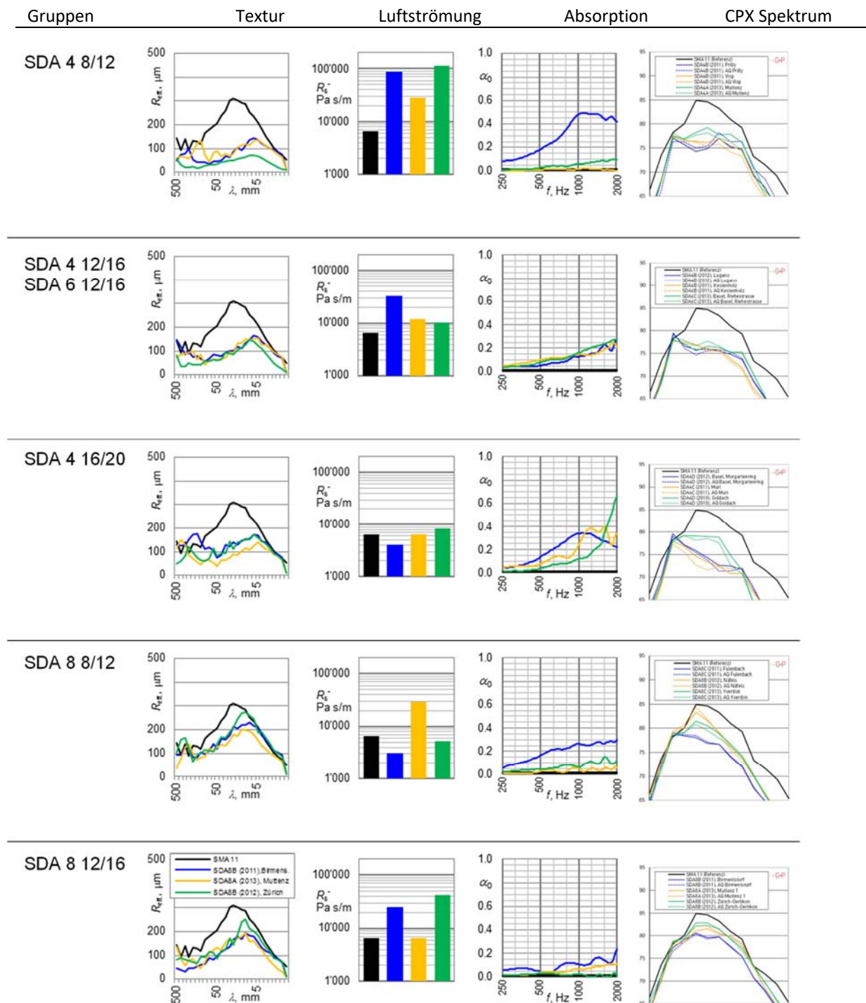
Abbildung 37: Textur-, Luftströmung-, Absorption- und CPX-Daten kategorisiert nach Belagsklasse und Hohlraumgehalt.
