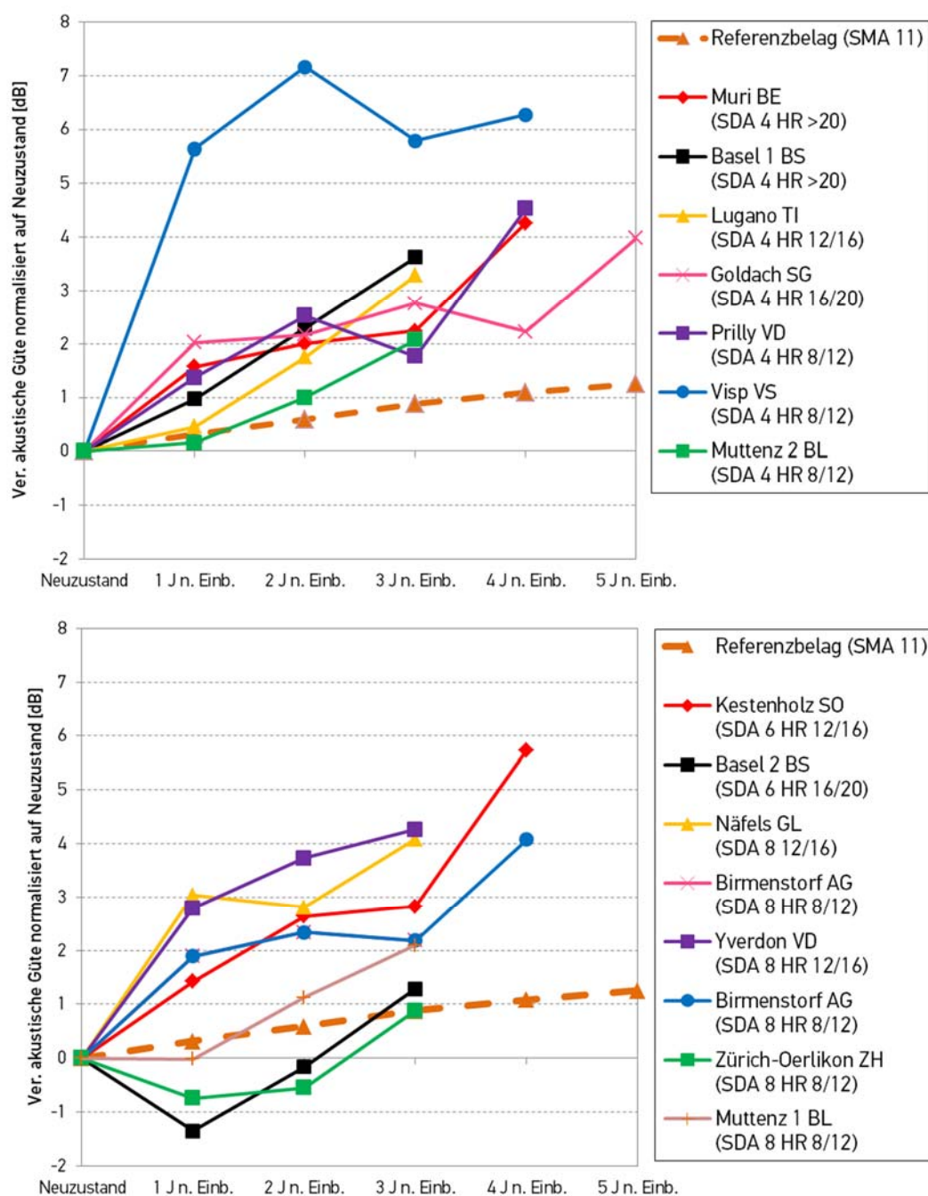
Abbildung 19: Veränderung der akustischen Güte seit Einbau (Streckenmittelwerte CPX PW) normalisiert auf Neuzustand im Vergleich zu einem konventionellen dichten Belag SMA 11 als Referenz (orange).
