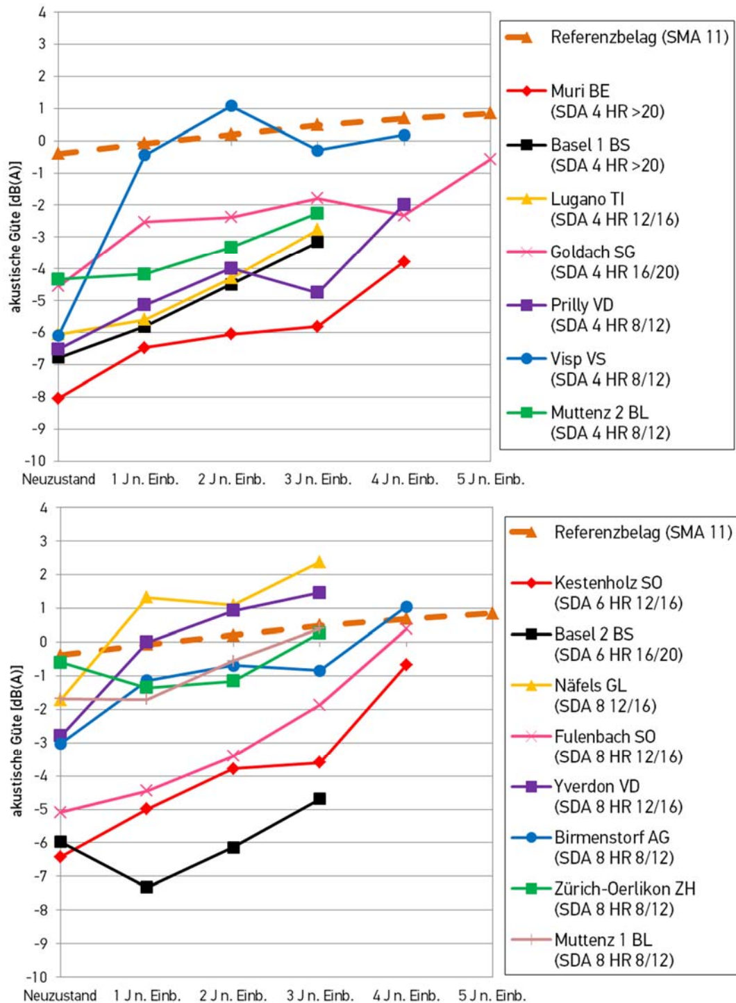
Abbildung 18: Veränderung der akustischen Güte seit Einbau (Streckenmittelwerte CPX PW) im Vergleich zu einem konventionellen dichten Belag SMA 11 als Referenz (orange).
