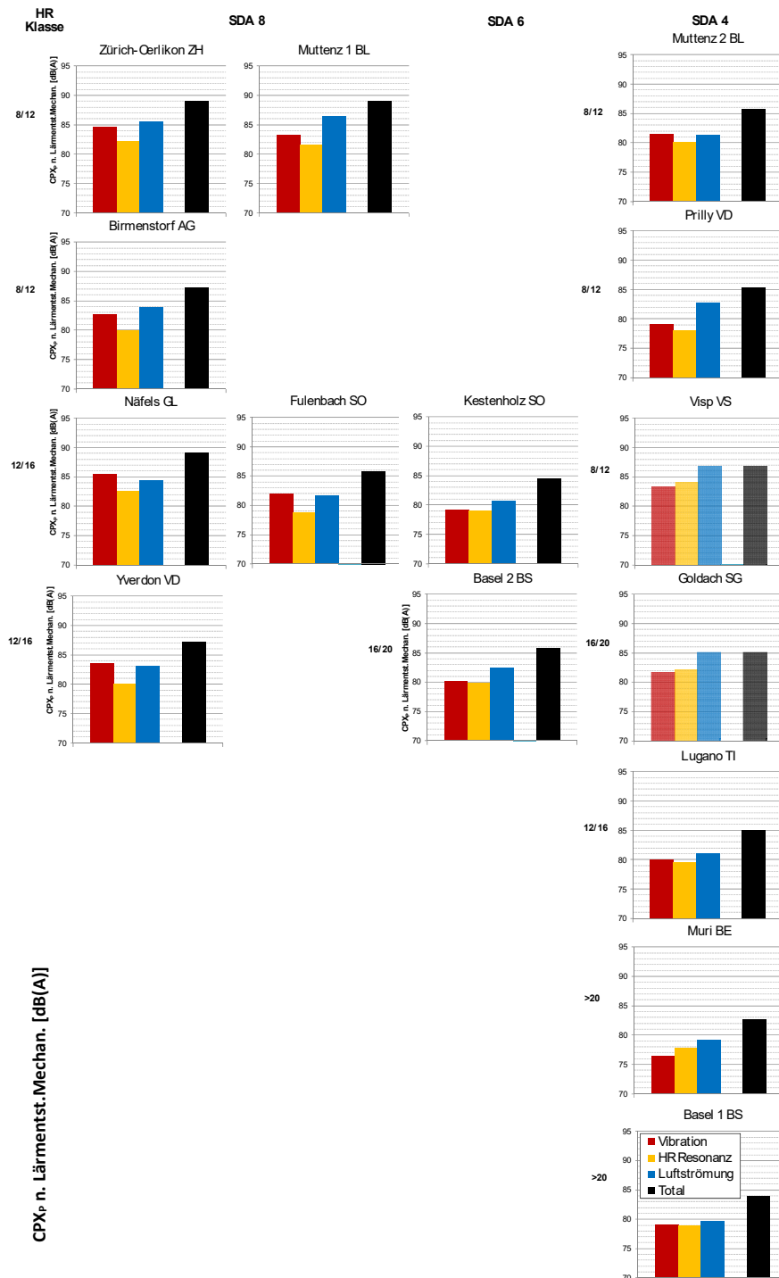
Abbildung 14: Rollgeräusch pro Lärmestehungsart aufgrund Wirkungsanalyse Schallentstehung (siehe Anhang A 3) im Neuzustand. Bemerkung: Für die Beläge in Goldach und Visp liegen für den Neuzustand keine Wirkungsanalysen vor, deshalb wird für diese Beläge der Zustand nach einem Jahr gezeigt.
