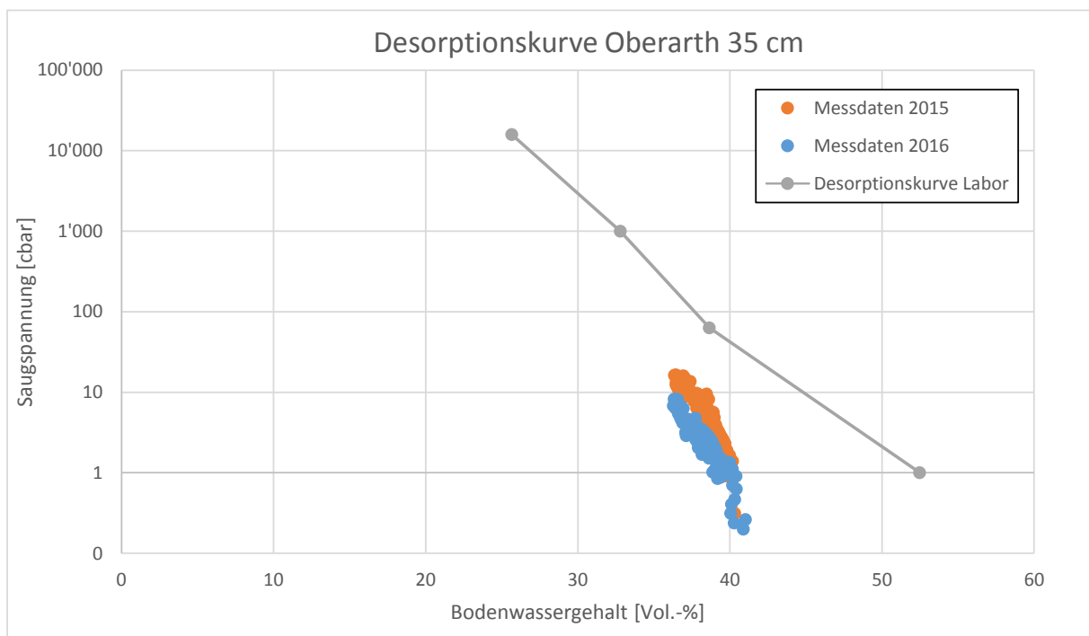
Abbildung 16: Desorptionskurve Oberarth mit den im Labor und im Feld bestimmten Messwert
