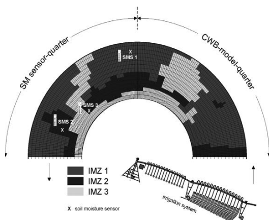
Abbildung 35: Darstellung einer teilflächenspezifischen Beregnung
