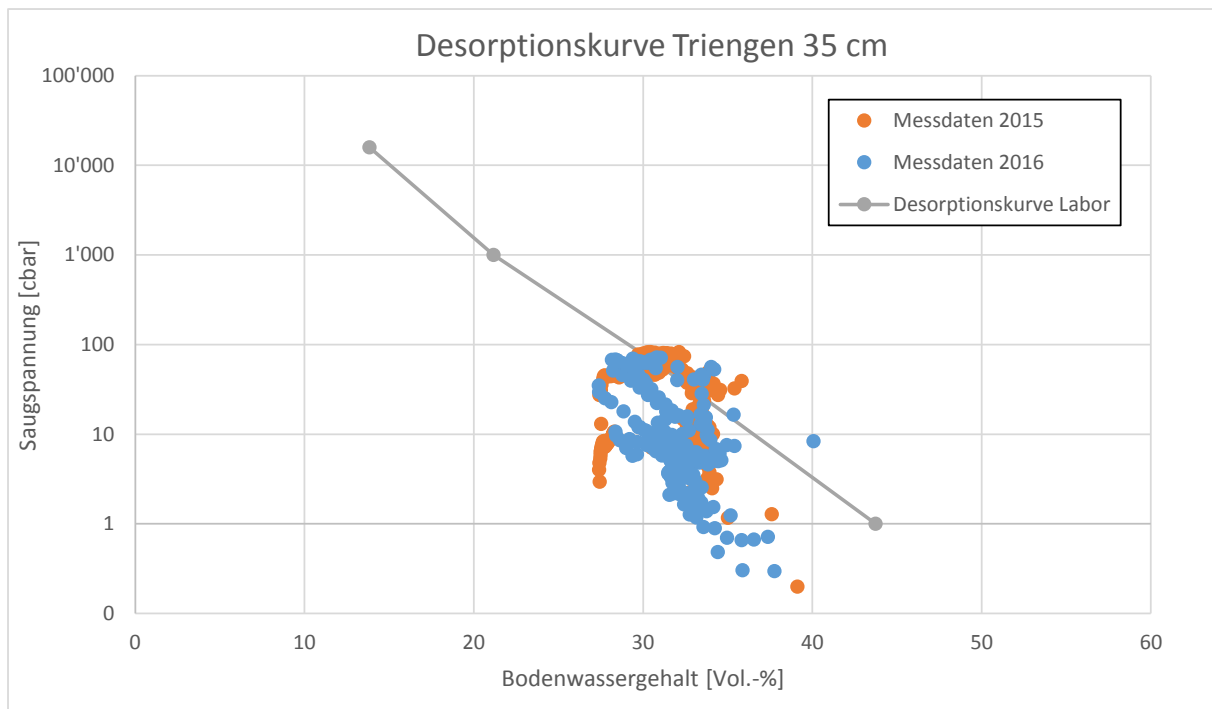
Abbildung 15: Desorptionskurve Triengen mit den im Labor und im Feld bestimmten Messwerten
