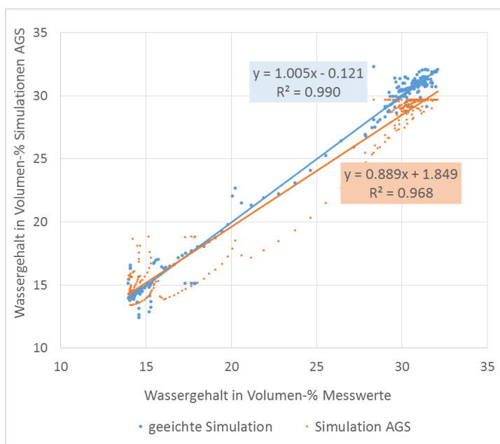
Abbildung 28: Korrelationsgraphik: Mittelwert der Trime-Sonden Messwerte in 20 cm und 35 cm Tiefe korreliert mit «Simulation AGS» (rote Punkte) und «geeichter Simulation» (blaue Punkte) für die Periode Januar bis Oktober 2015 in Gelfingen
