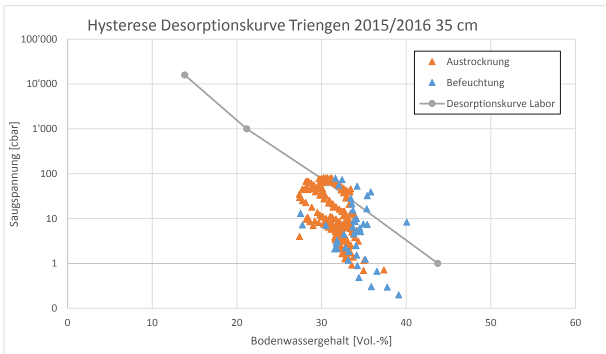
Abbildung 17: Desorptionskurve Triengen 2015/2016 Einfluss der Hysterese
