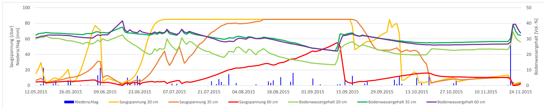
Abbildung 21: Tagesmittel-Zeitreihe Saugspannung und Niederschlag (linke y-Achse) und Bodenwassergehalt (rechte y-Achse) in Triengen 2015 (12.05. – 24.11.2015)
