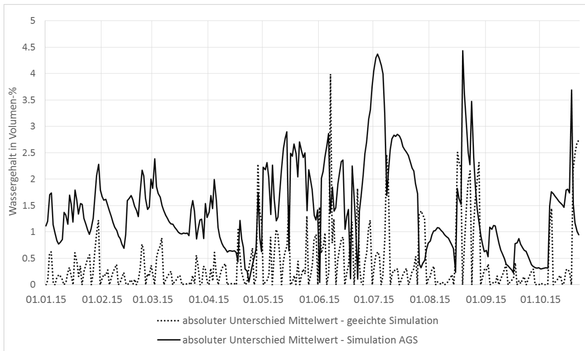
Abbildung 29: Abweichungen der «Simulation AGS» und der «geeichten Simulation» von den Messwerten als absolute Differenzen zum gemessenen Mittelwert der Trime-Sonden in 20 cm und 35 cm Tiefe von Januar bis Oktober 2015
