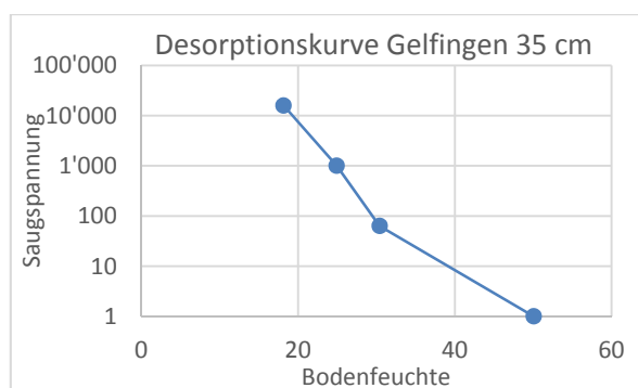
Abbildung 9: Desorptionskurve in 35 cm Tiefe
