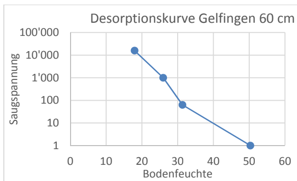
Abbildung 10: Desorptionskurve in 60 cm Tiefe
