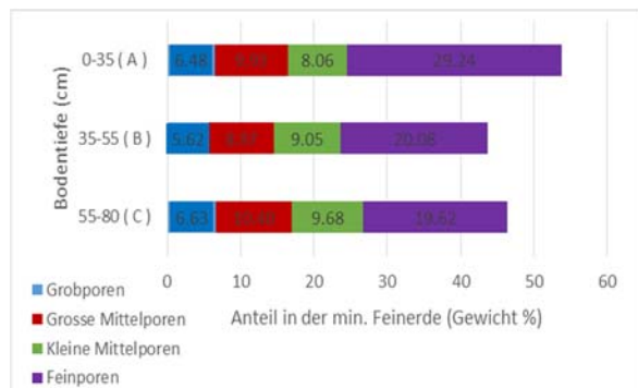
Abbildung 7: Porengrößenverteilung
