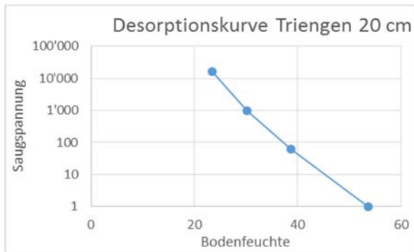
Abbildung 8: Desorptionskurve in 20 cm Tiefe
