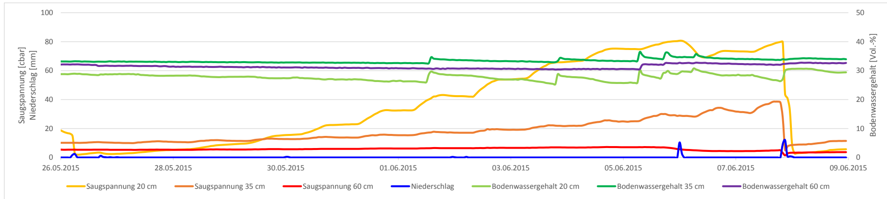
Abbildung 23: Bewässerungseffekt in den Bodenfeuchtemessungen Triengen 2015 (26.05. - 09.06.2015)
