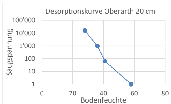
Abbildung 8: Desorptionskurve in 20 cm Tiefe
