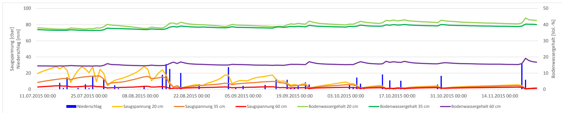
Abbildung 24: Tagesmittel-Zeitreihe Saugspannung und Niederschlag (linke y-Achse) und Bodenwassergehalt (rechte y-Achse) in Oberarth 2015 (11.07. - 24.11.2015)
