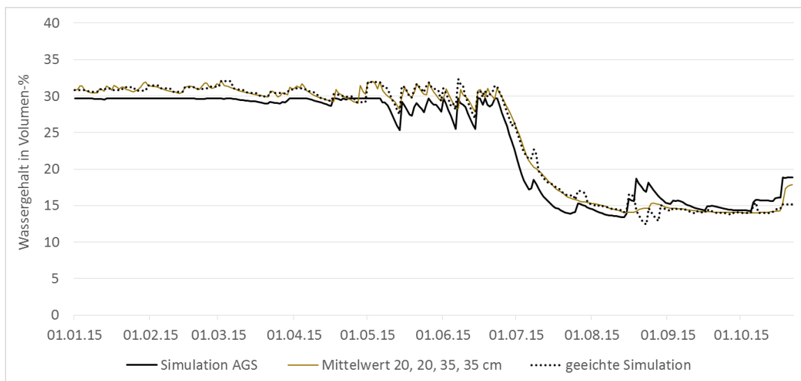
Abbildung 27: Bodenfeuchte in Gelfingen: Verlauf der «Simulation AGS» und der «geeichten Simulation» im Vergleich mit den Messwerten (Mittelwert der Trime-Sonden in 20 cm und 35 cm Tiefe) von Januar bis Oktober 2015
