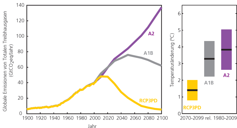
Abbildung 1: Klimaszenarien und Temperaturänderung in der Schweiz im 21. Jahrhundert
