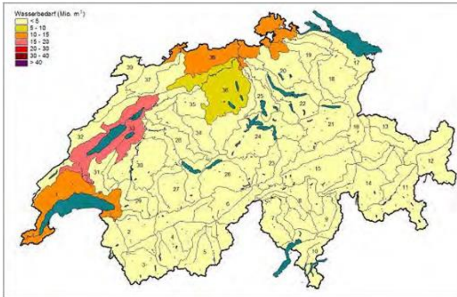
Abbildung 3: Mittlerer jährlicher Bewässerungsbedarf in der Schweizer Landwirtschaft für die Periode 1981-2010
