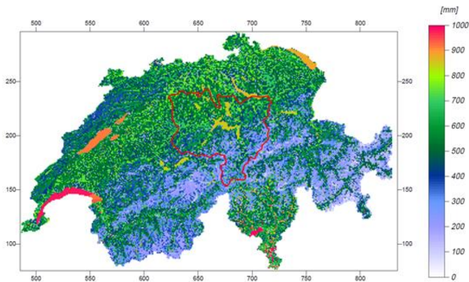
Abbildung 8: Mittlere Jahresverdunstung der Schweiz von 1973-1992 in mm.
