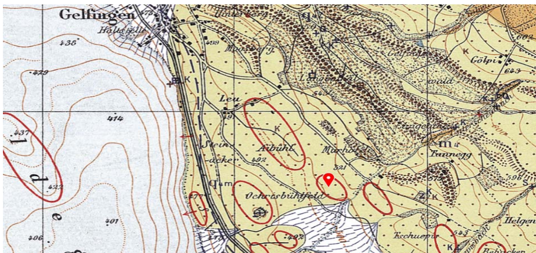
Abbildung 3: Geologischer Atlas der Schweiz 3 (rot umrandet: Drumlin, gepunktete Linie: Moränenwall, hellbraun: Moräne)
