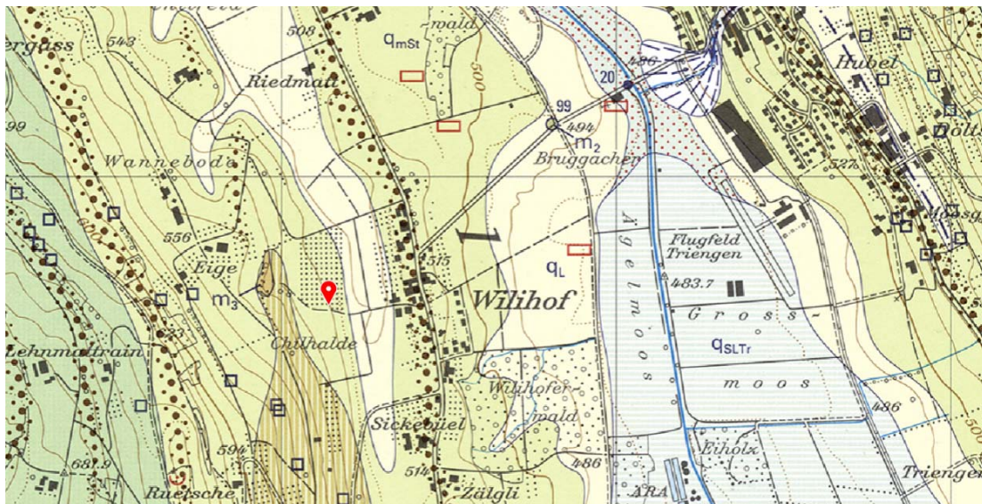
Abbildung 3: Geologischer Atlas der Schweiz 3 (hellbraun: Schwemmlehm, grün: Moräne, blau: Seesedimente)
