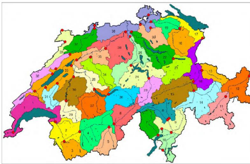
Abbildung 2: Die 39 Regionen der Schweiz mit Abflussstationen
