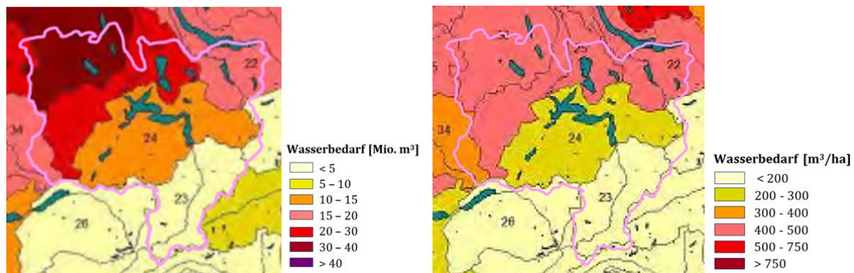
Abbildung 9: Ausschnitt Zentralschweiz: Potentieller Bewässerungsbedarf im Jahr 2003
