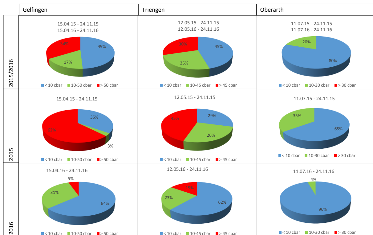
Abbildung 18: Saugspannungswerte 2015 und 2016: blau: feucht, grün: optimal, rot: trocken, bewässerungsbedürftig. Die Messdaten stammen von der für die jeweilige Kultur optimalen Messtiefe (Äpfel 35 cm, Kirschen 35 cm, Heidelbeeren 20 cm). Aufgrund der unterschiedlichen Messbeginne unterscheiden sich die Zeitperioden der verschiedenen Kulturen. Sie wurden aber für die verschiedenen Jahre jeweils identisch gewählt.
