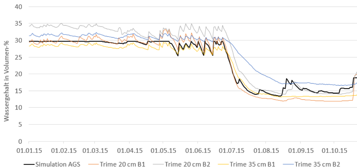
Abbildung 26: Bodenfeuchte in Gelfingen: Vergleich der «Simulation AGS» mit den Messwerten in 20 cm und 35 cm Tiefe von Januar bis Oktober 2015
