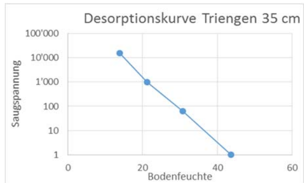
Abbildung 9: Desorptionskurve in 35 cm Tiefe
