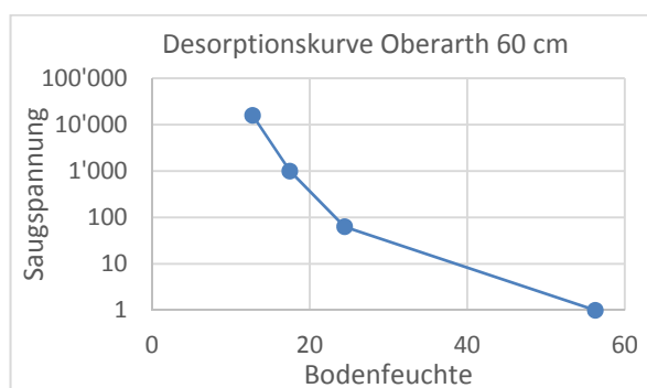
Abbildung 10: Desorptionskurve in 60 cm Tiefe
