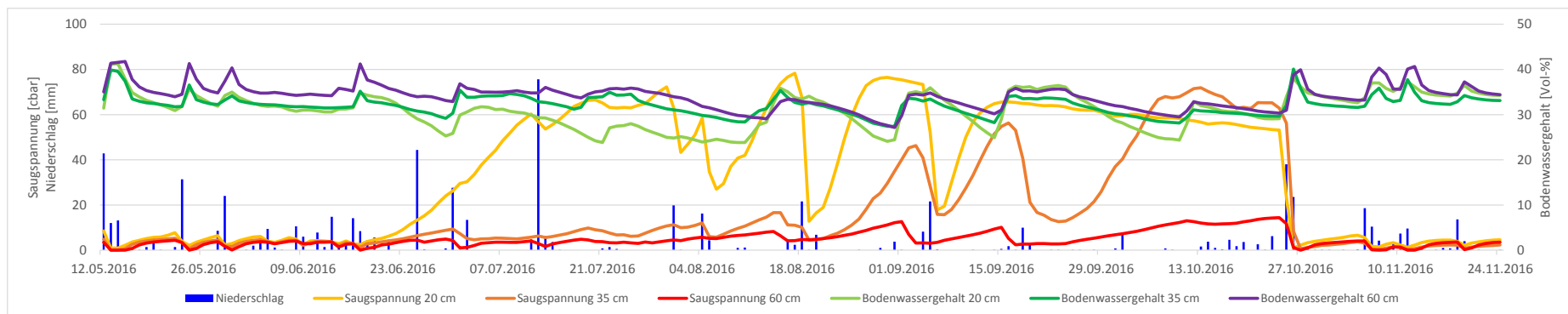
Abbildung 22: Tagesmittel-Zeitreihe Saugspannung und Niederschlag (linke y-Achse) und Bodenwassergehalt (rechte y-Achse) in Triengen 2016 (12.05. – 24.11.2016)
