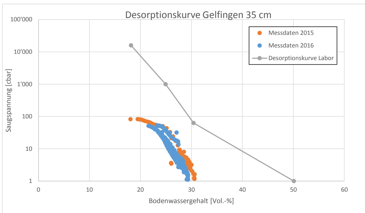
Abbildung 14: Desorptionskurve Gelfingen mit den im Labor und im Feld bestimmten Messwerten
