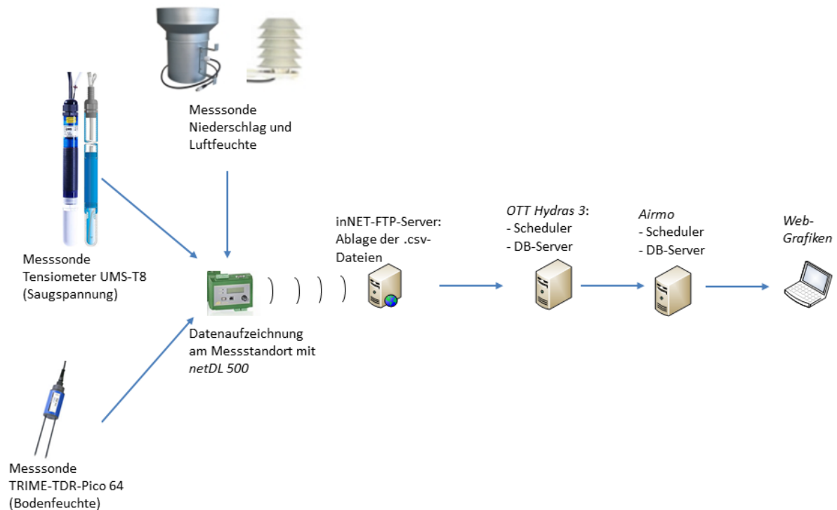
Abbildung 12: Schematische Darstellung Messeinrichtungen und Datenkommunikation
