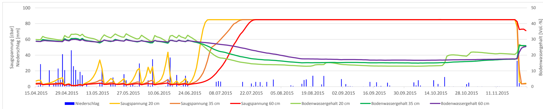
Abbildung 19: Tagesmittel-Zeitreihe Saugspannung und Niederschlag (linke y-Achse) und Bodenwassergehalt (rechte y-Achse) in Gelfingen 2015 (15.04. - 24.11.2015)
