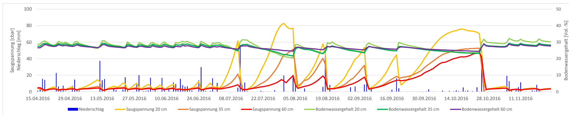
Abbildung 20: Tagesmittel-Zeitreihe Saugspannung und Niederschlag (linke y-Achse) und Bodenwassergehalt (rechte y-Achse) in Gelfingen 2016 (15.04. - 24.11.2016)
