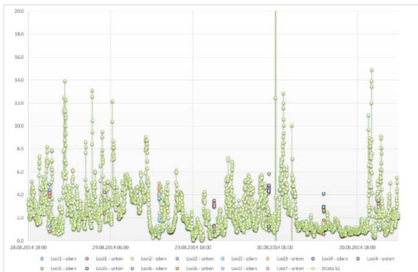
Abbildung 10: Zeitreihe der \text{NH}_3 Konzentration des miniDOAS und der Impingersysteme (Witzwil 28.-30. August 2014). Für die Impingersysteme ist der Mittelpunkt der jeweils 8-stündigen Messintervalle angegeben.
