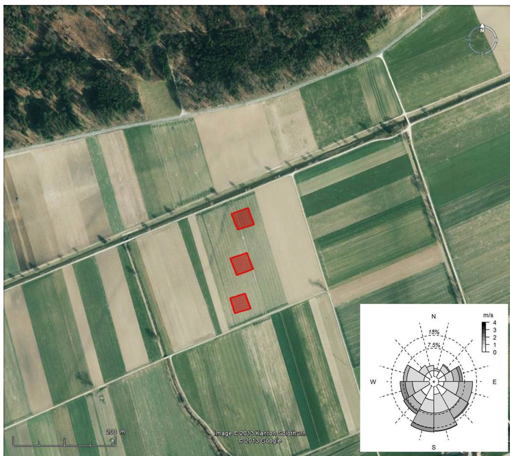
Abbildung A.53: Anordnung der Versuchspartzen. Die Windrosengrafik zeigt die Frequenz der Windrichtung, sowie die dazugehörigen Windgeschwindigkeiten (in m/s) auf 1 m über Boden, welche über die gesamte Versuchsdauer gemessen wurden.
