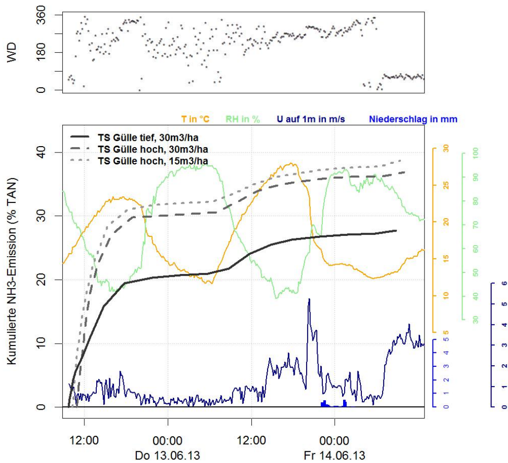
Abbildung A.59: Gemessener Verlauf der kumulierten Emission sowie die gemittelten Meteorparameter Lufttemperatur (T) und relative Luftfeuchte (RH) und die vor Ort gemessene Windgeschwindigkeit (U) und Windrichtung (WD).
