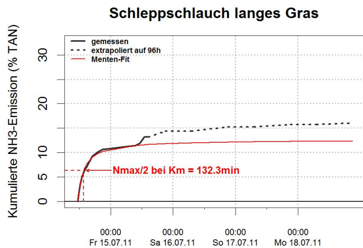
Abbildung A.32: Verlauf der kumulierten NH 3 -Emission. Die Grafiken zeigen die gemessenen und extrapolierten Emissionsverläufe, sowie die gefitteten Verläufe nach Michaelis-Menten.
