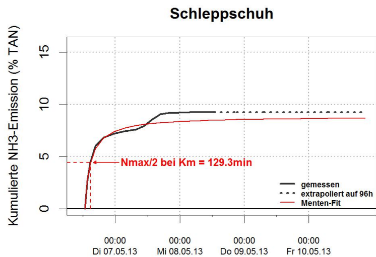
Abbildung A.28: Verlauf der kumulierten NH 3 -Emission. Die Grafiken zeigen die gemessenen und extrapolierten Emissionsverläufe, sowie die gefitteten Verläufe nach Michaelis-Menten.
