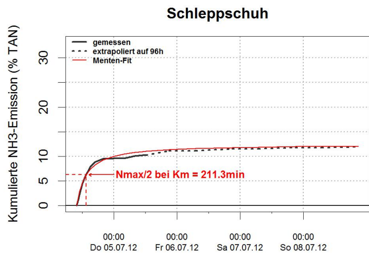
Abbildung A.16: Verlauf der kumulierten NH 3 -Emission. Die Grafiken zeigen die gemessenen und extrapolierten Emissionsverläufe, sowie die gefitteten Verläufe nach Michaelis-Menten.
