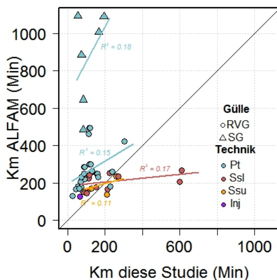
Abbildung 39: Vergleich der gefundenen Km-Werte mit den prognostizierten Werten des Modelles ALFAM (Søgaard et al., 2002). RVG: Rindviehgülle; SG: Schweinegülle; Pt: Prallteller; Ssl: Schleppschlauch; Ssu: Schleppschuh; Inj: Gölledrill.
