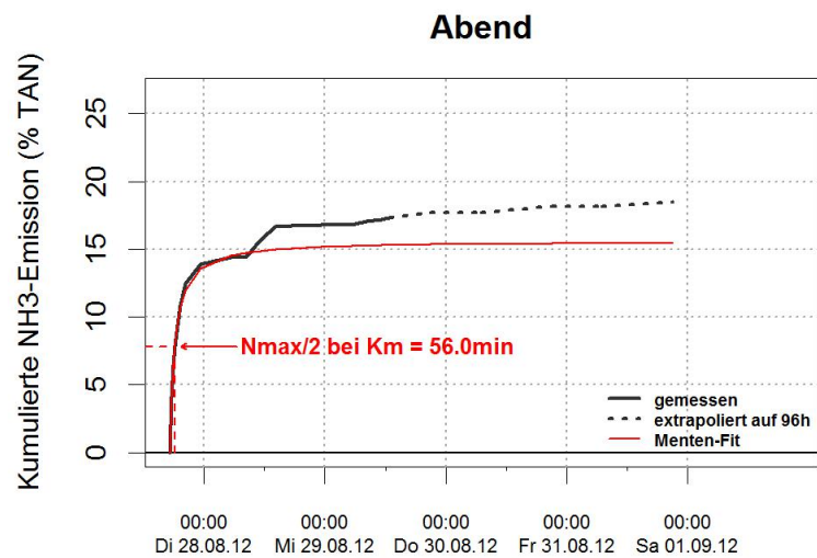
Abbildung A.40: Verlauf der kumulierten NH 3 -Emission. Die Grafiken zeigen die gemessenen und extrapolierten Emissionsverläufe, sowie die gefitteten Verläufe nach Michaelis-Menten.
