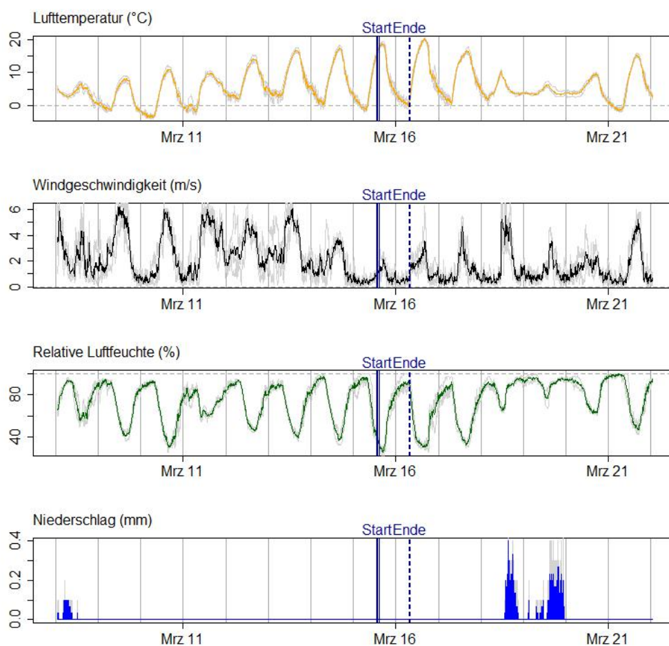
Abbildung A.46: Aufzeichnung der Wetterstationen Bern / Zollikofen, Grenchen (SO) und Koppigen (BE). Die Grafik zeigt die gemittelten Werte der Lufttemperatur (°C), Windgeschwindigkeit (m/s), relativen Luftfeuchte (%), sowie der 10-minütigen Niederschlagssumme (mm). Hellgrau eingezeichnet sind die effektiv gemessenen Werte der einzelnen Stationen. Start und Ende des Versuches sind zusätzlich in der Grafik eingetragen.
