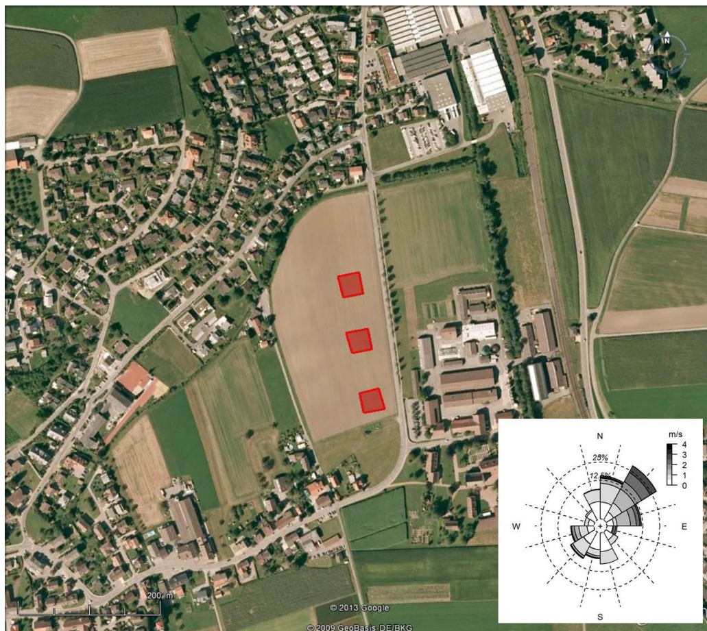
Abbildung A.41: Anordnung der Versuchspartzellen. Die Windrosengrafik zeigt die Frequenz der Windrichtung, sowie die dazugehörigen Windgeschwindigkeiten (in m/s) auf 1 m über Boden, welche über die gesamte Versuchsdauer gemessen wurden.
