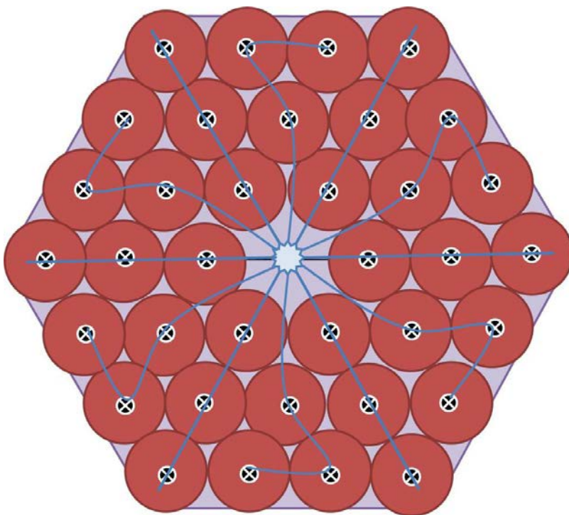
Abbildung 14: Geometrische Anordnung der Düsen der künstlichen Quelle.
