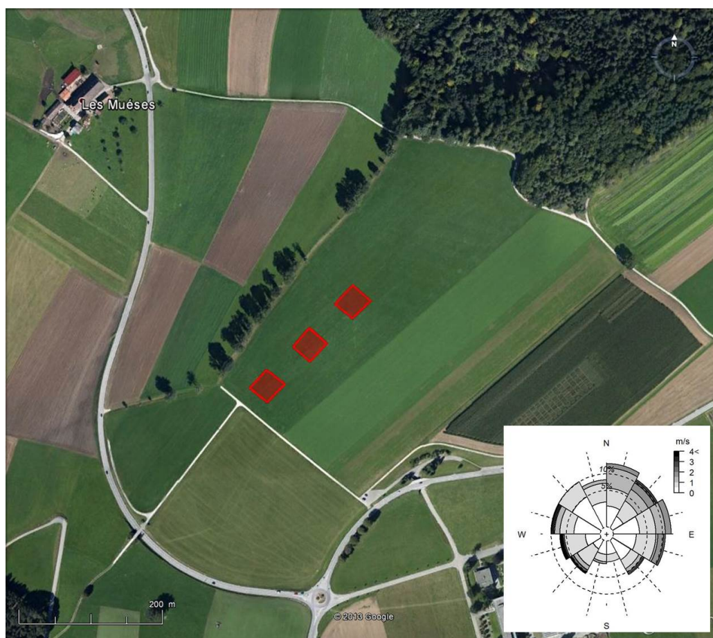
Abbildung A.13: Anordnung der Versuchspartzellen. Die Windrosengrafik zeigt die Frequenz der Windrichtung, sowie die dazugehörigen Windgeschwindigkeiten (in m/s) auf 1 m über Boden, welche über die gesamte Versuchsdauer gemessen wurden.
