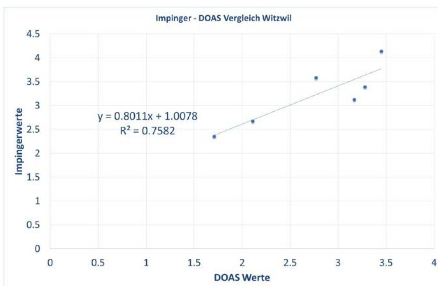
Abbildung 11: Regression der \text{NH}_3 Mittelwerte der 7 LOCI-Systeme mit den mittleren \text{NH}_3 miniDOAS Werten.
