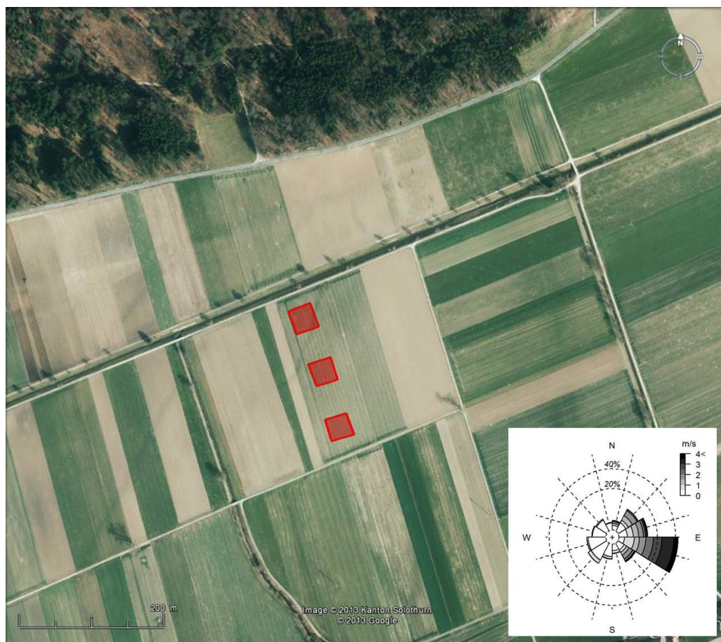
Abbildung A.61: Anordnung der Versuchsparzellen. Die Windrosengrafik zeigt die Frequenz der Windrichtung, sowie die dazugehörigen Windgeschwindigkeiten (in m/s) auf 1 m über Boden, welche über die gesamte Versuchsdauer gemessen wurden.
