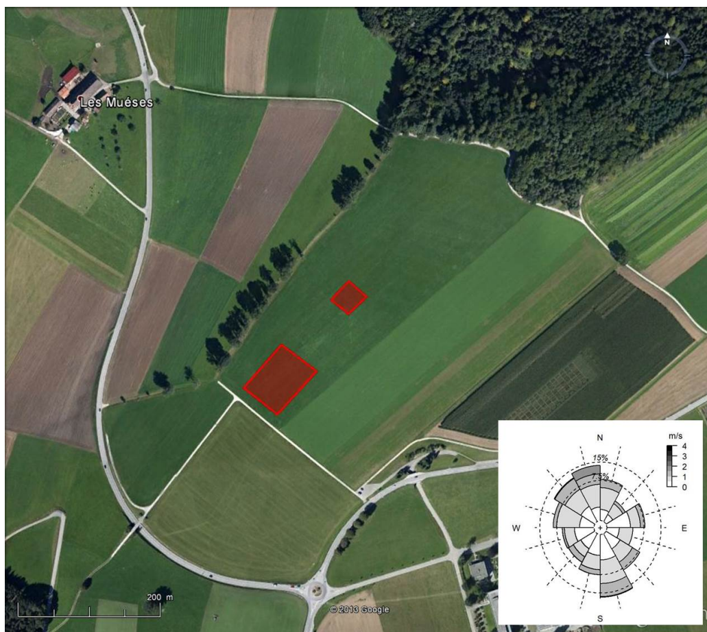
Abbildung A.5: Anordnung der Versuchspartzellen. Die Windrosengrafik zeigt die Frequenz der Windrichtung, sowie die dazugehörigen Windgeschwindigkeiten (in m/s) auf 1 m über Boden, welche über die gesamte Versuchsdauer gemessen wurden.
