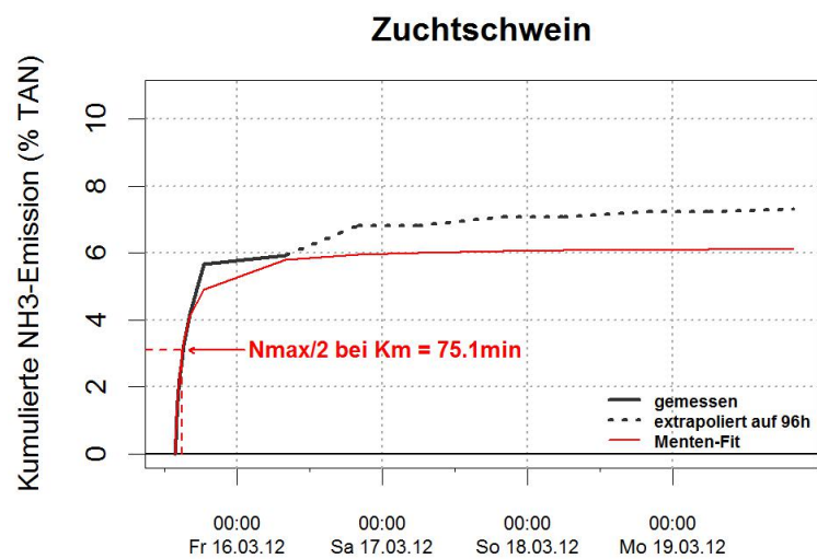
Abbildung A.48: Verlauf der kumulierten NH 3 -Emission. Die Grafiken zeigen die gemessenen und extrapolierten Emissionsverläufe, sowie die gefitteten Verläufe nach Michaelis-Menten.
