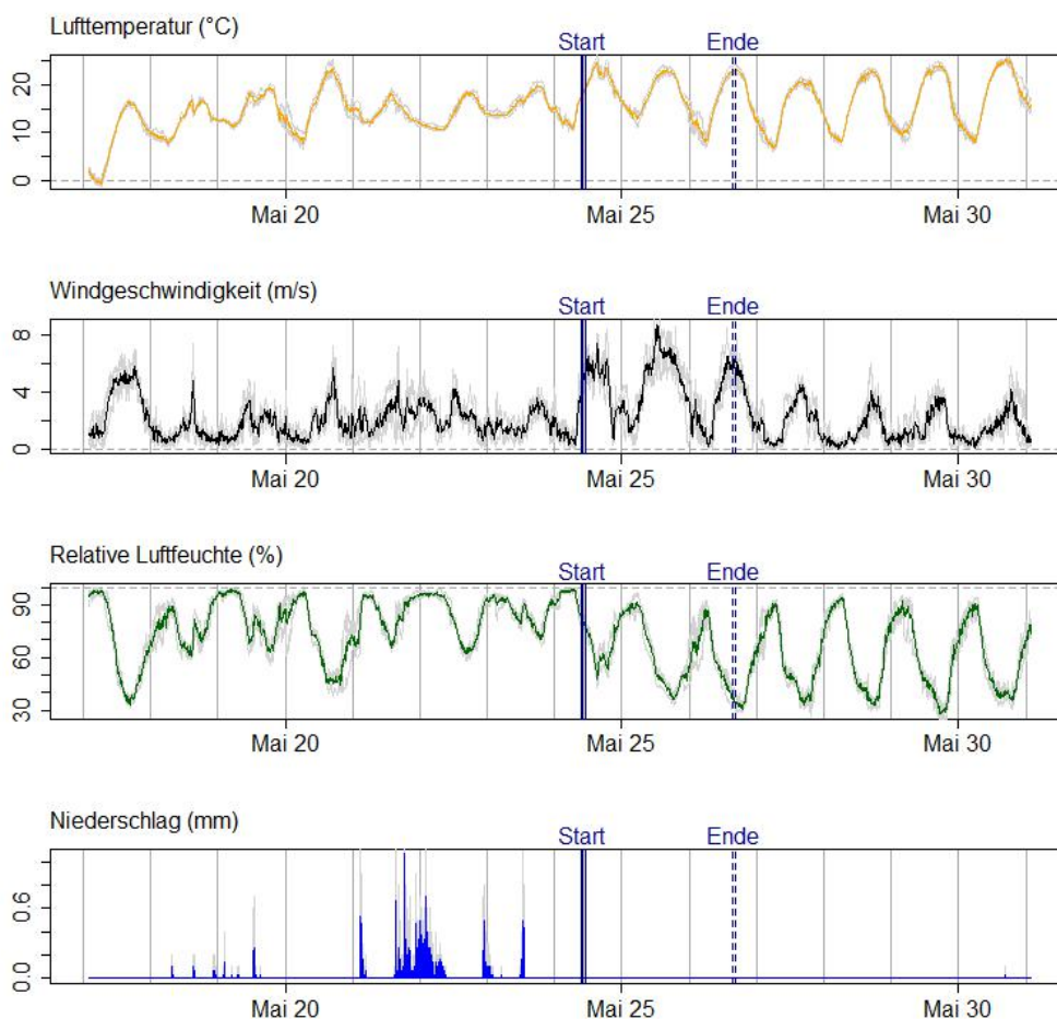
Abbildung A.50: Aufzeichnung der Wetterstationen Bern / Zollikofen, Grenchen (SO) und Koppigen (BE). Die Grafik zeigt die gemittelten Werte der Lufttemperatur (°C), Windgeschwindigkeit (m/s), relativen Luftfeuchte (%), sowie der 10-minütigen Niederschlagssumme (mm). Hellgrau eingezeichnet sind die effektiv gemessenen Werte der einzelnen Stationen. Start und Ende des Versuches sind zusätzlich in der Grafik eingetragen.
