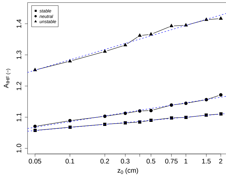
Abbildung C.2: A_{IHF} für X = 20\text{m} , drei Stabilitätsregime und verschiedene z_0 mittels WindTrax; Profilberechnungen wie für ZINST 2013 (siehe Kapitel B.4 ).
