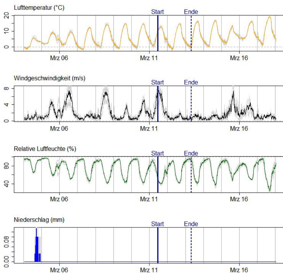
Abbildung A.66: Aufzeichnung der Wetterstationen Bern / Zollikofen, Grenchen (SO) und Koppigen (BE). Die Grafik zeigt die gemittelten Werte der Lufttemperatur (°C), Windgeschwindigkeit (m/s), relativen Luftfeuchte (%), sowie der 10-minütigen Niederschlagssumme (mm). Hellgrau eingezeichnet sind die effektiv gemessenen Werte der einzelnen Stationen. Start und Ende des Versuches sind zusätzlich in der Grafik eingetragen.
