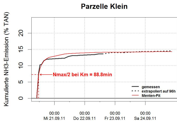
Abbildung A.36: Verlauf der kumulierten NH 3 -Emission. Die Grafiken zeigen die gemessenen und extrapolierten Emissionsverläufe, sowie die gefitteten Verläufe nach Michaelis-Menten.
