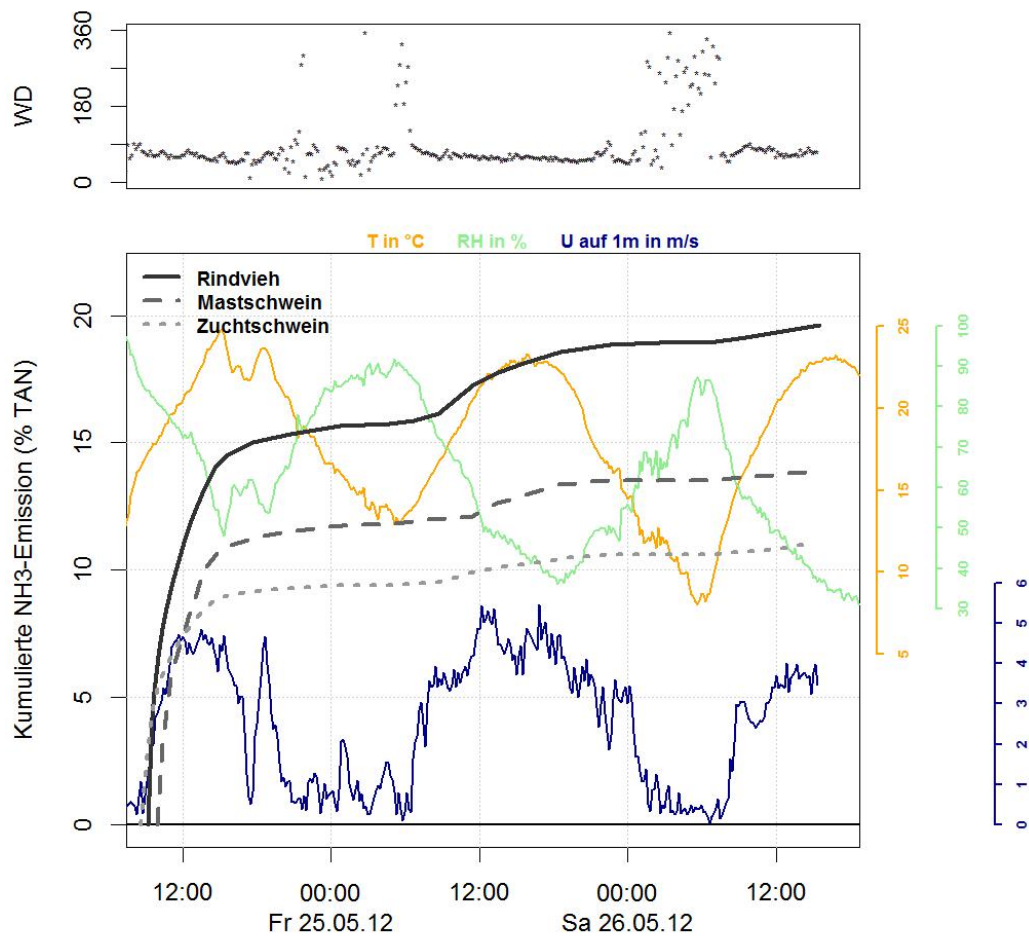
Abbildung A.51: Gemessener Verlauf der kumulierten Emission sowie die gemittelten Meteorparameter Lufttemperatur (T) und relative Luftfeuchte (RH) und die vor Ort gemessene Windgeschwindigkeit (U) und Windrichtung (WD).
