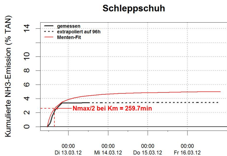
Abbildung A.12: Verlauf der kumulierten NH 3 -Emission. Die Grafiken zeigen die gemessenen und extrapolierten Emissionsverläufe, sowie die gefitteten Verläufe nach Michaelis-Menten.
