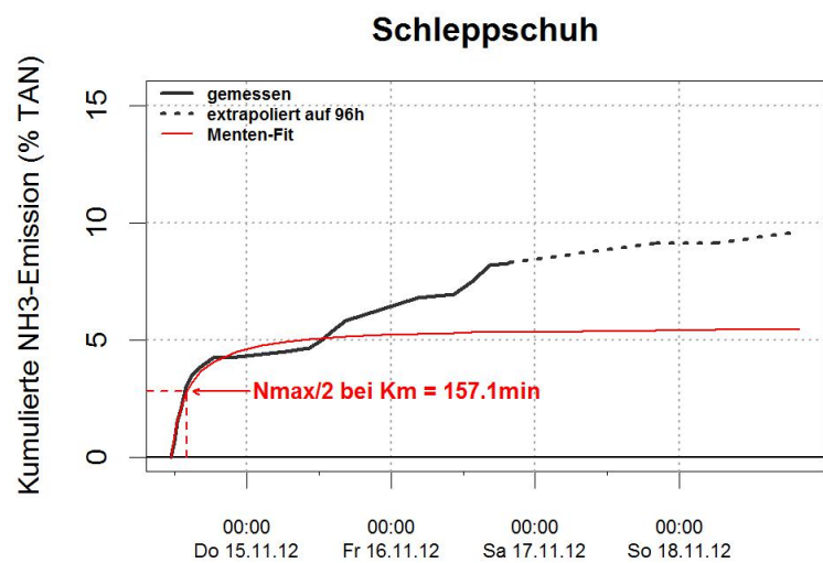
Abbildung A.24: Verlauf der kumulierten NH 3 -Emission. Die Grafiken zeigen die gemessenen und extrapolierten Emissionsverläufe, sowie die gefitteten Verläufe nach Michaelis-Menten.
