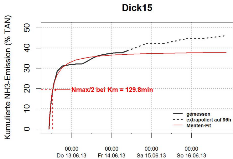
Abbildung A.60: Verlauf der kumulierten NH 3 -Emission. Die Grafiken zeigen die gemessenen und extrapolierten Emissionsverläufe, sowie die gefitteten Verläufe nach Michaelis-Menten.
