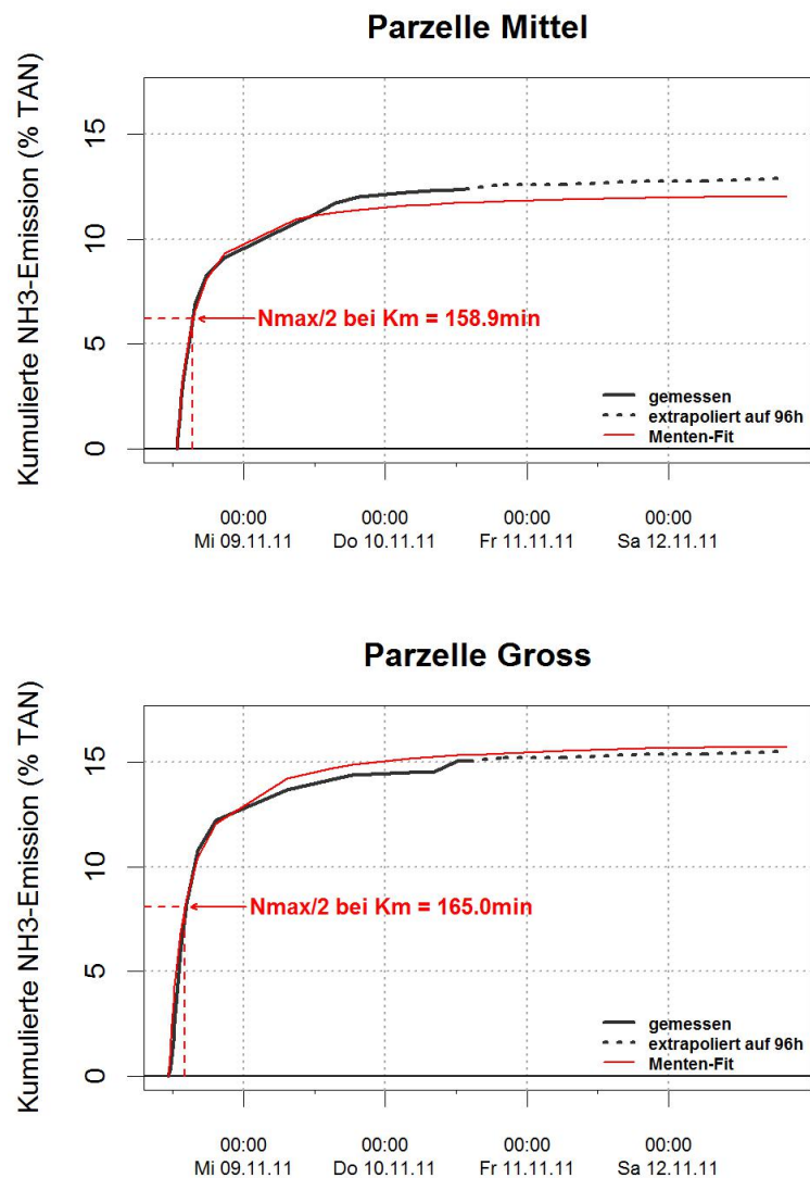
Abbildung A.8: Verlauf der kumulierten \text{NH}_3 -Emission. Die Grafiken zeigen die gemessenen und extrapolierten Emissionsverläufe, sowie die gefitteten Verläufe nach Michaelis-Menten.
