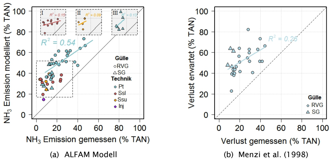
Abbildung 38: Vergleich der bestehenden Messreihe mit den NH 3 -Emissionsmodellen ALFAM (Søgaard et al., 2002) und Menzi et al. (1998). RVG: Rindviehgülle; SG: Schweinegülle; Pt: Prallteller; Ssl: Schleppschlauch; Ssu: Schleppschuh; Inj: Gölledrill. ALFAM Subplots: I) RVG/Ssl, II) RVG/Ssu, III) SG/Pt.
