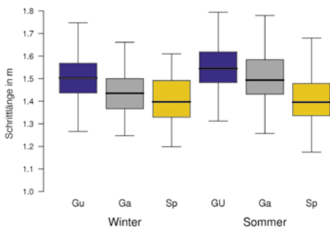
Abb. 15: Schrittweiten auf den verschiedenen Bodenarten (Gu: planbefestigter Boden mit Gummibelag; Ga: Gussasphalt; Sp: Betonspaltenboden) bei den Erhebungen im Winter und Sommer.
