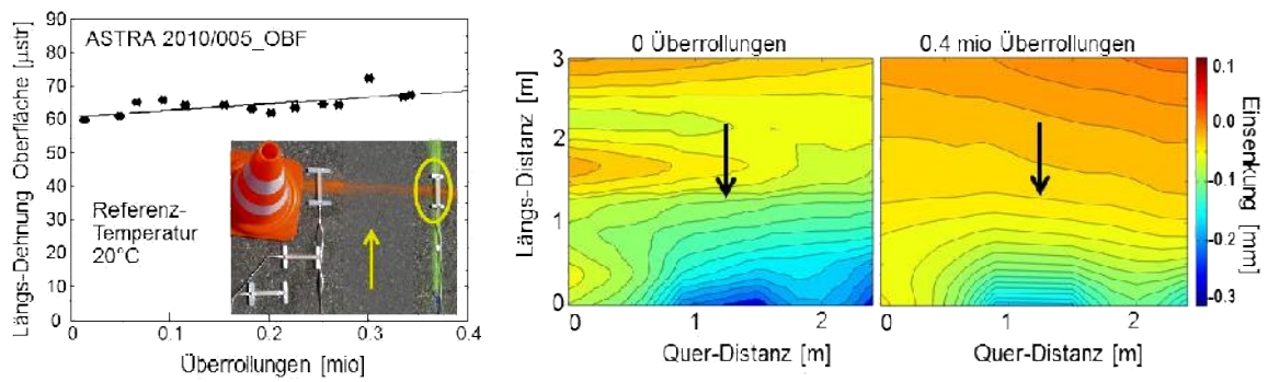
Bild 2: Dehnungsamplituden vs. Überrollungen Bild 3: Einsenkungen mit ETH-Delta gemessen
