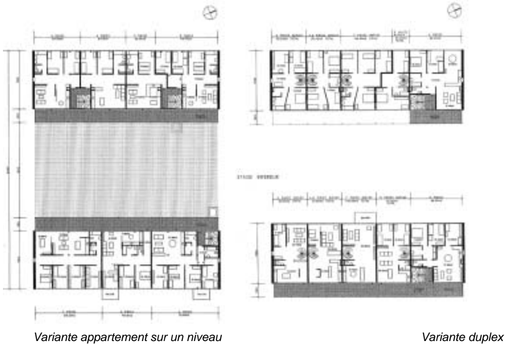
Figure 7 : Evolution du projet des Ouches : variantes
