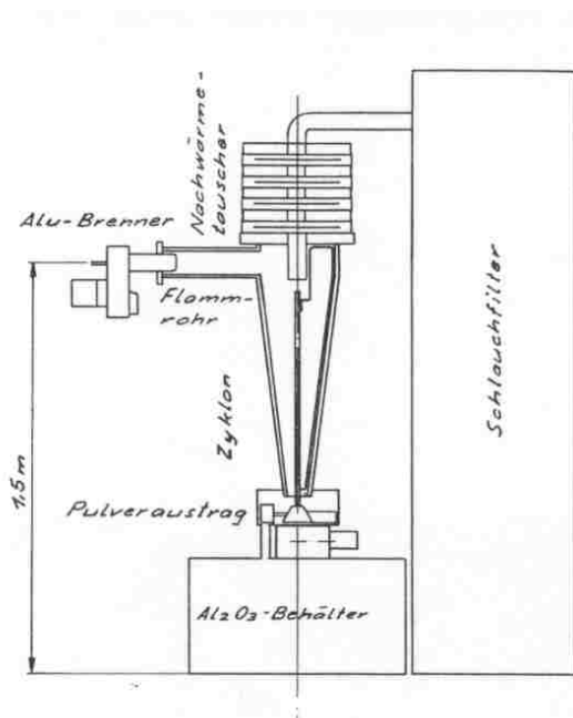
Bild 3a: offene Gesamtanlage 1988
