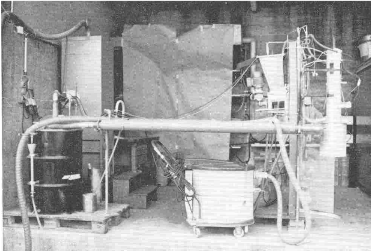
Bild 3a: offene Gesamtanlage 1988
