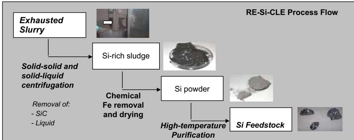
Figur 3: Prozesskette zur Rezyklierung von Silizium (Bildquelle HCT Shaping Systems)
