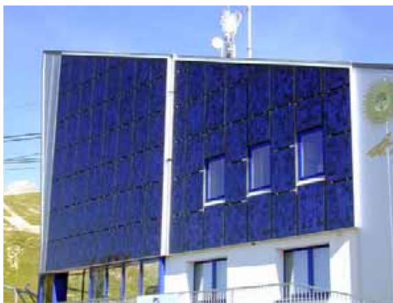
Figur 26: 9.7 kWp Fassade 'Piz Nair Talstation' (Bildquelle NET)
