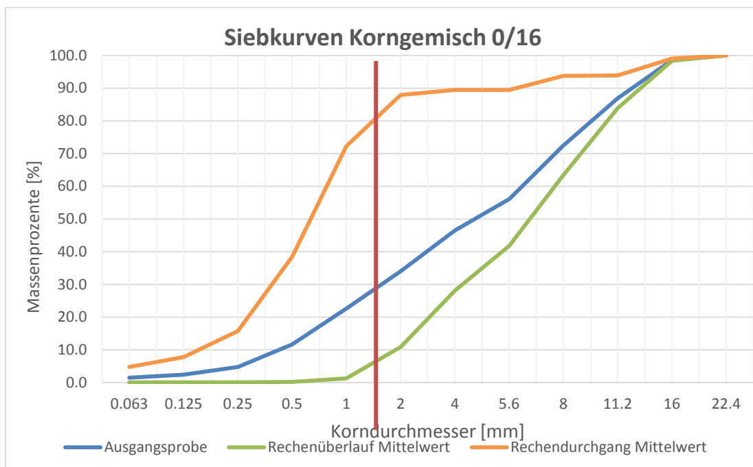
Abbildung 27: Siebkurve Feldversuch Mühlbach: Korngemisch 0/16
