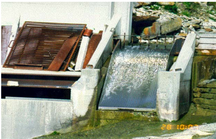
Abbildung 4: Pilotprojekt Coanda-Rechen am Rappierbach bei Hinterrhein GR. Erster Coanda-Rechen in der Schweiz. Inbetriebnahme 1998
