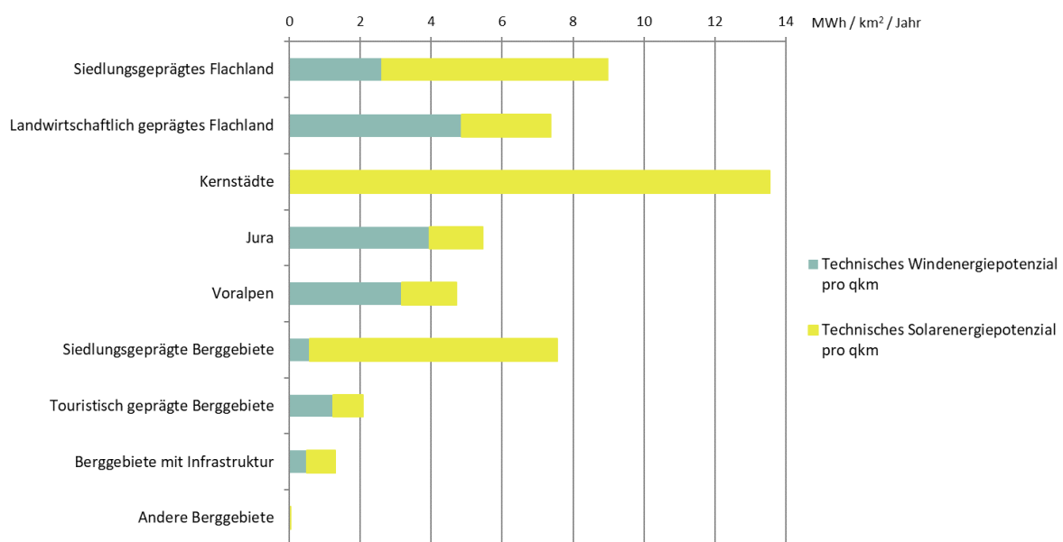
Abb. 22: Technisches Energiepotenzial pro km² in den Charakterlandschaften in MWh pro Jahr.
